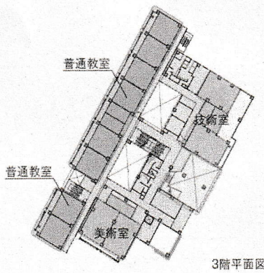
3階平面図
