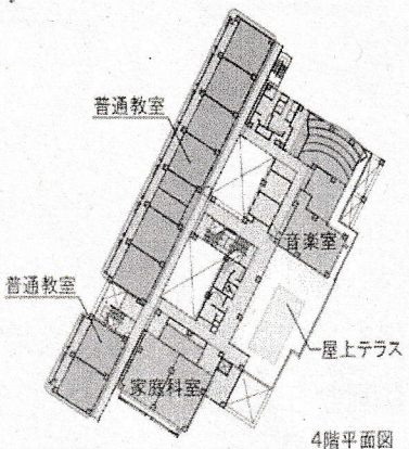
4階平面図
