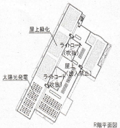
R階平面図
